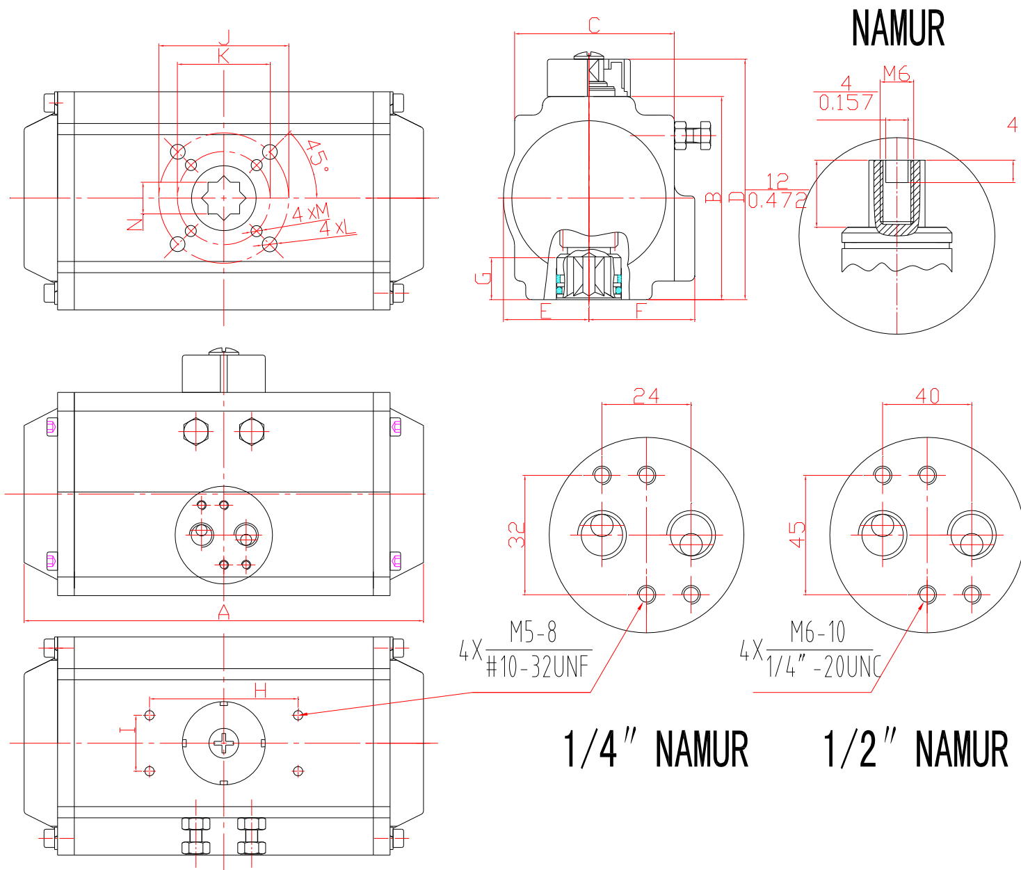
AT 型气动执行器外型尺寸及连接尺寸示意图
